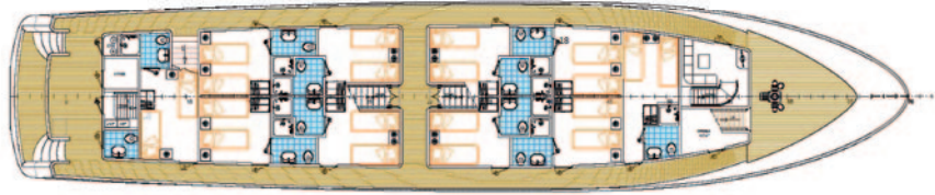
CUBIERTA PRINCIPAL
